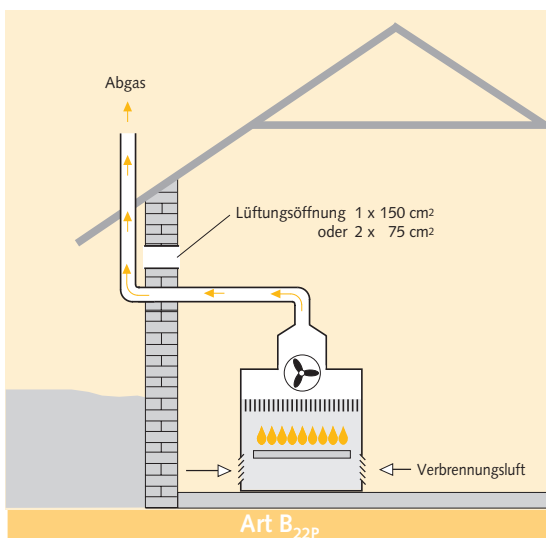
Bild 21: Raumluftabhängiges Gasgerät ohne Strömungssicherung mit Gebläse hinter dem Wärmetauscher; Abgasabfuhrung mit Überdruck ohne besondere Dichtheitsanforderung, deshalb Lüftungsöffnung erforderlich.
