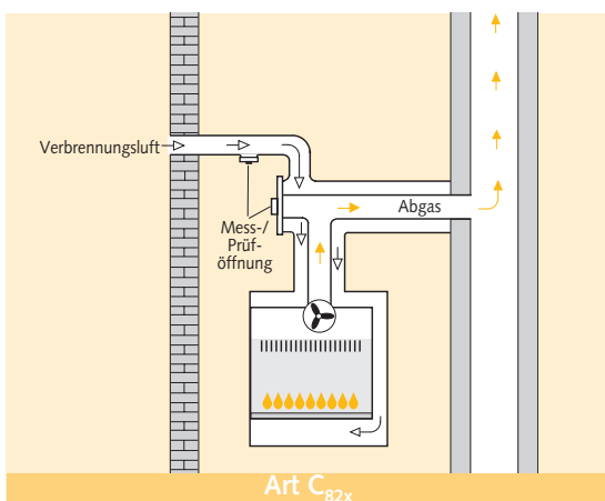
Bild 35: Raumluftunabhängiges Gasgerät mit Gebläse hinter dem Wärmetauscher; auch Gasgerät Art C 8 3x möglich; getrennte Verbrennungsluftzuführung aus dem Freien; gemeinsame Abgasanlage im Unterdruckbetrieb; alle unter Überdruck stehenden Teile des Abgasweges sind verbrennungsluftumspült, Mehrfachbelegung möglich (z. B. Gas-Kombitherme).
