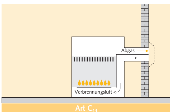
Bild 25: Raumluftunabhängiges Gasgerät ohne Gebläse; Mündungen für Verbrennungsluftzu- und Abgasabführung im gleichen Druckbereich (z. B. Außenwand-Raumheizer)
