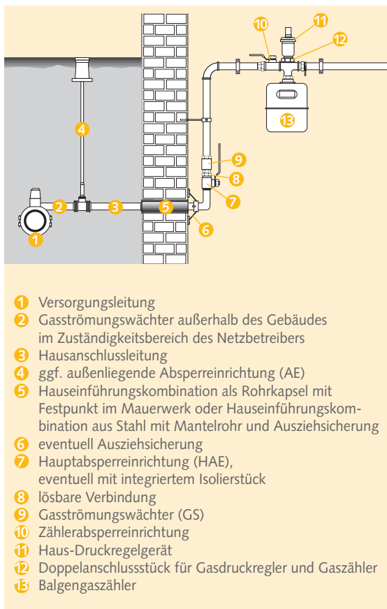
Bild 8: Beispiel für einen Erdgas-Hausanschluss mit Regler-/Zählerverbindung
