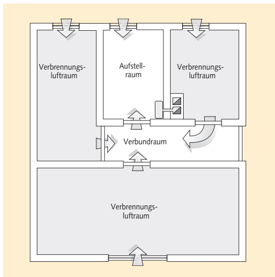
Bild 44: Mittelbarer Verbrennungsluftverbund
