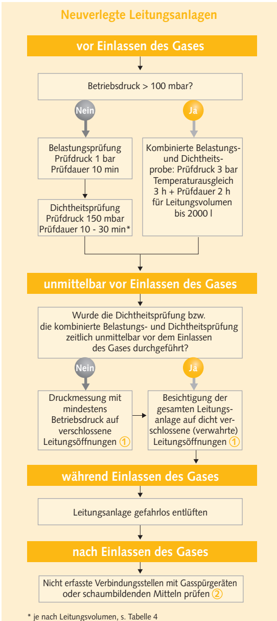
Bild 13: Vorgehensweise beim Einlassen von Gas in neuverlegte Leitungsanlagen
