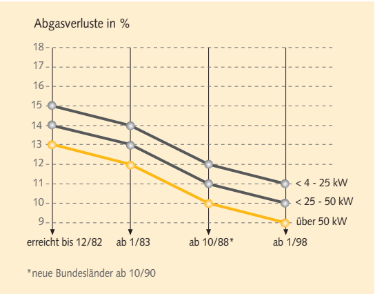
Bild 53: Höchstzulässige Abgasverluste von Gas- und Ölf Feuerungsanlagen in Prozent
