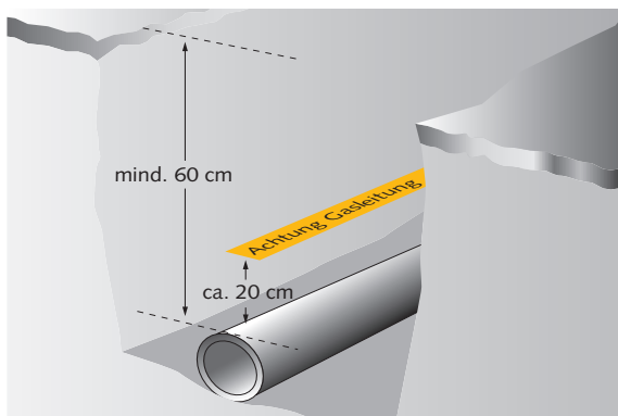
Bild 7: Erdverlegte Außenleitung
