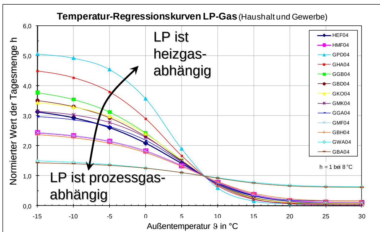
Abbildung 10 Darstellung der Temperaturabhängigkeit der einzelnen Lastprofiltypen Sigmoid-Profile nach TUM in der Ausprägung 04
