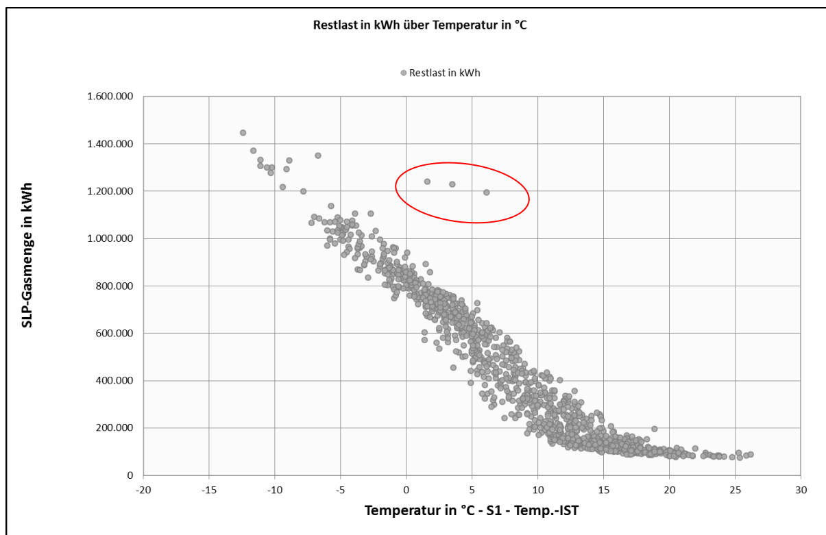
Abbildung 22 Restlastpunktwolke in Abhängigkeit zu der Tagesmitteltemperatur mit Datenfehler
