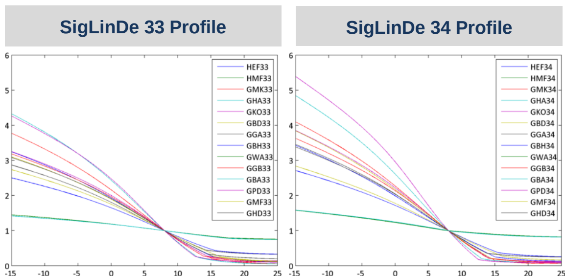
Abbildung 11 Darstellung der Temperaturabhängigkeit der einzelnen Lastprofiltypen SigLinDe-Profile nach FfE in der Ausprägung 33 und 34
