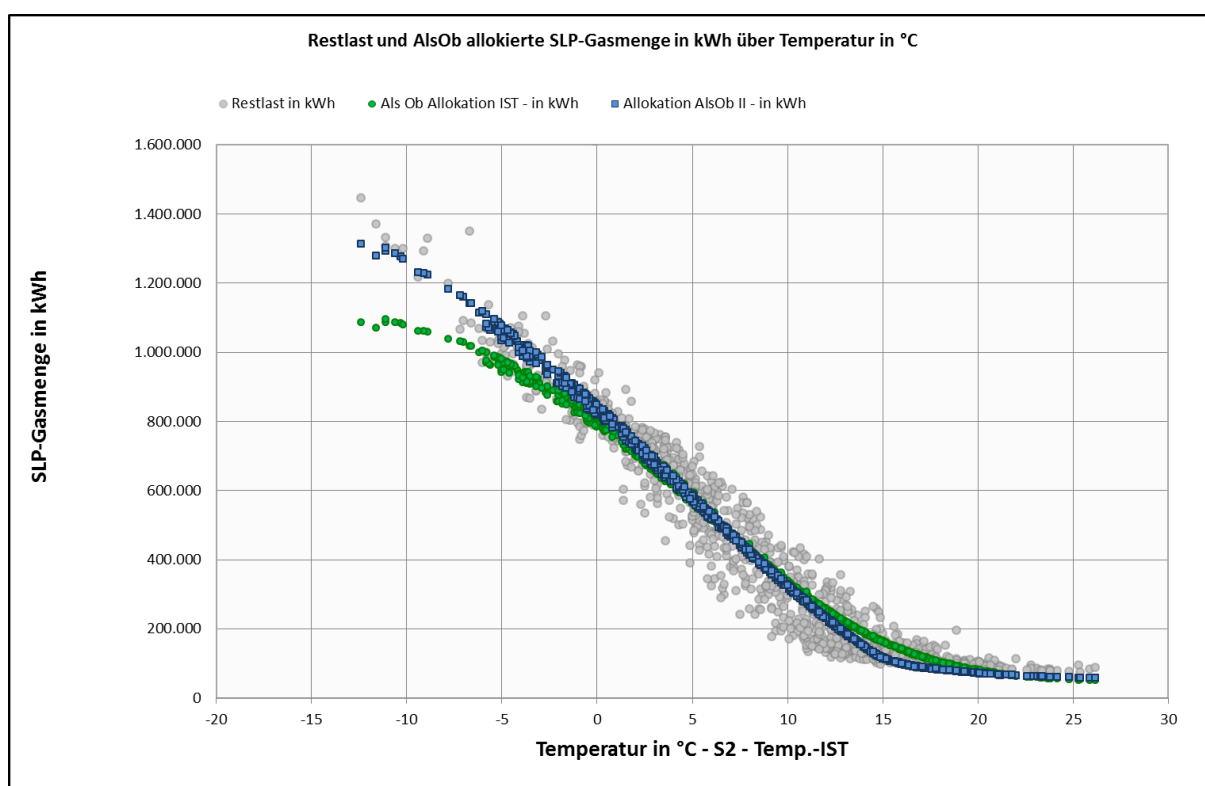
Abbildung 24 Darstellung Als-Ob Allokation SLP-Ausprägung „34“
