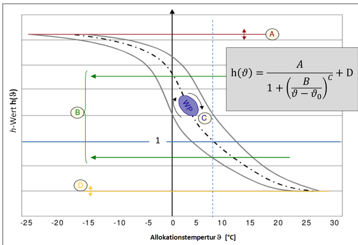
Abbildung 32 Wirkungsweise der Sigmoid-Funktion
