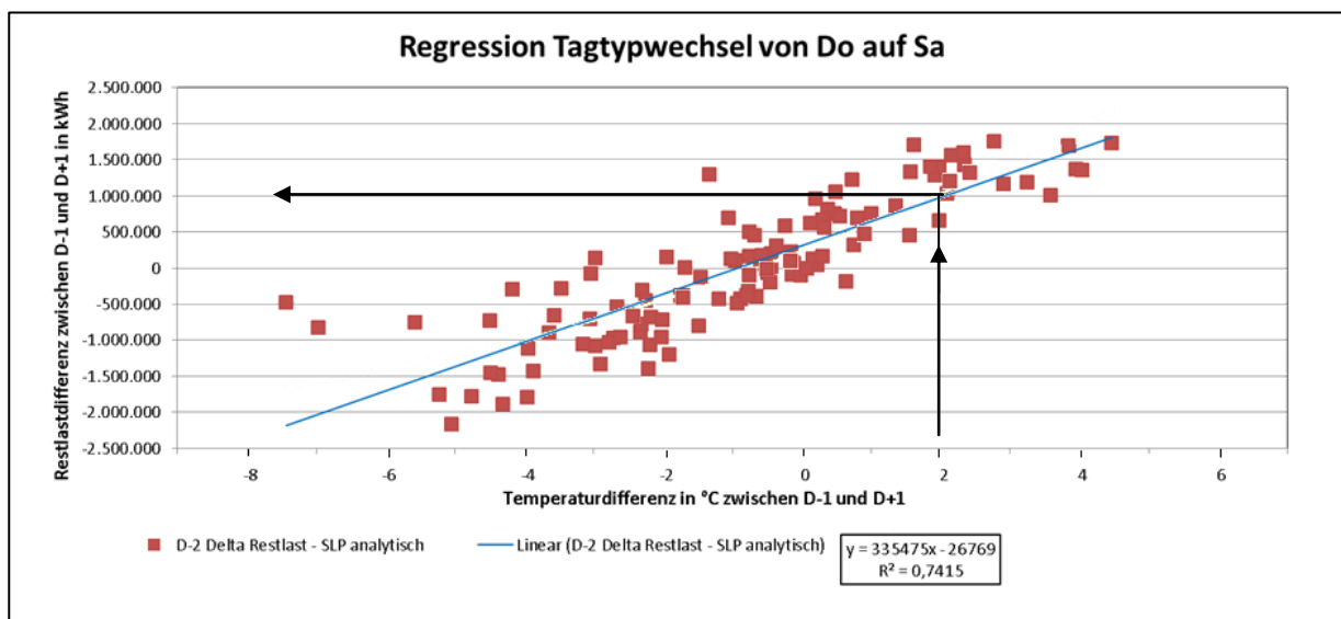
Abbildung 17 Anwendungsbeispiel für Regressionsgeraden nach Tagestypwechsel
