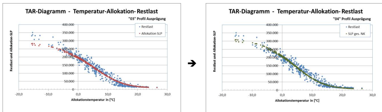
Abbildung 19 TAR-Diagramme zur Abbildung der Restlast und der Allokation über der Allokationstemperatur
