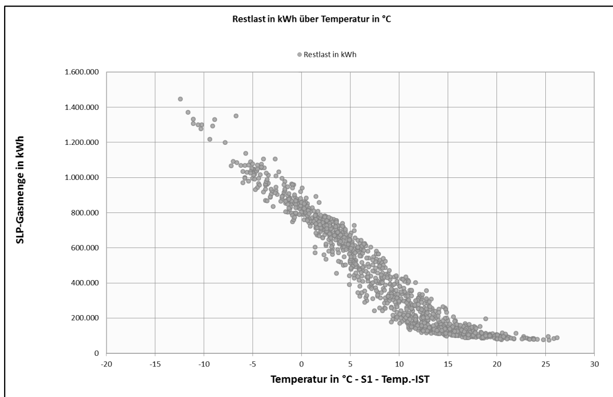
Abbildung 21 Restlastpunktwolke in Abhängigkeit zu der Tagesmitteltemperatur ohne Datenfehler
