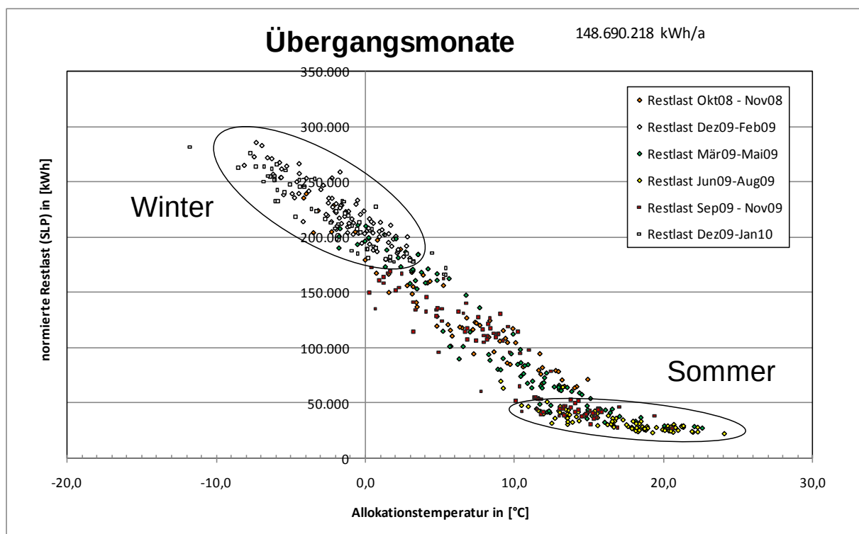
Abbildung 27 Darstellung der Restlastpunktwolke in den Übergangsmonaten
