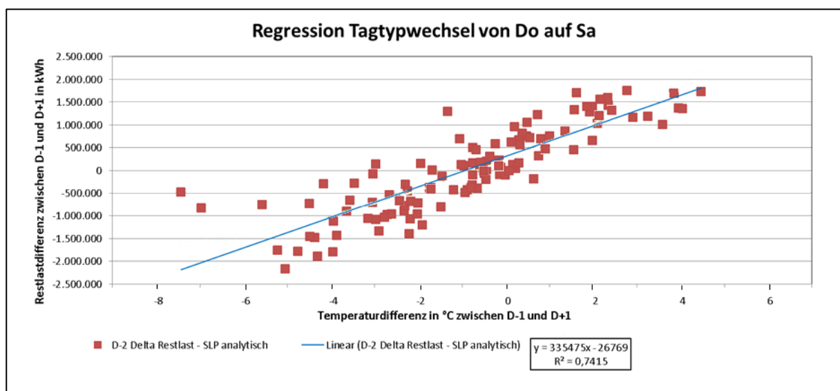
Abbildung 16 Beispiel für Regressionsgeraden nach Tagestypwechsel
