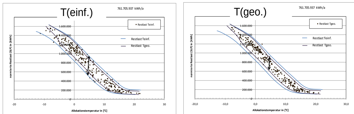
Abbildung 26 Vergleichende Darstellung einfache Tagesmitteltemperatur zur Mehrtages-Temperatur mit geometrischen Reihe
