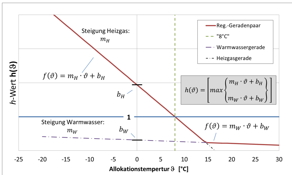
Abbildung 33 Wirkungsweise des Regressionsgeradenpaar
