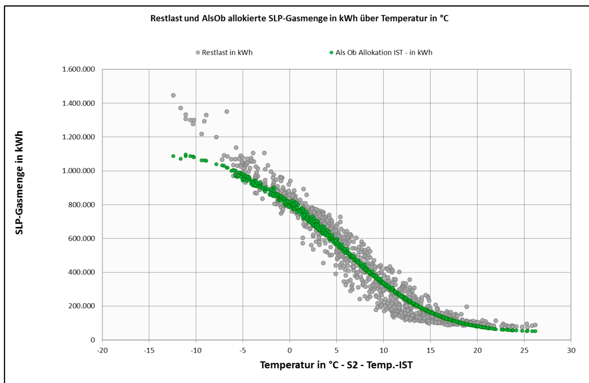
Abbildung 23 Darstellung ursprüngliche SLP-Ausprägung zur Restlast
