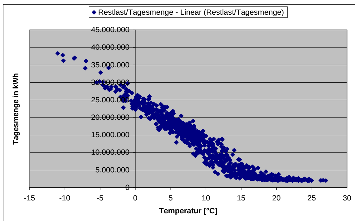
Abbildung 14 Beispiel für die Ermittlung einer Netzregressionsfunktion
