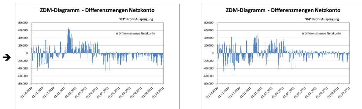
Abbildung 18 ZDM-Diagramme für Abbildung der Differenzmenge des Netzkontos (NK0)
